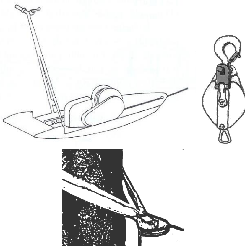
KMF con 100 m di fune da 6-8mm, due cinghie tubolari da 1000 kg lunghe 2,5-3 m e una carrucola apribile da 1000 kg.
