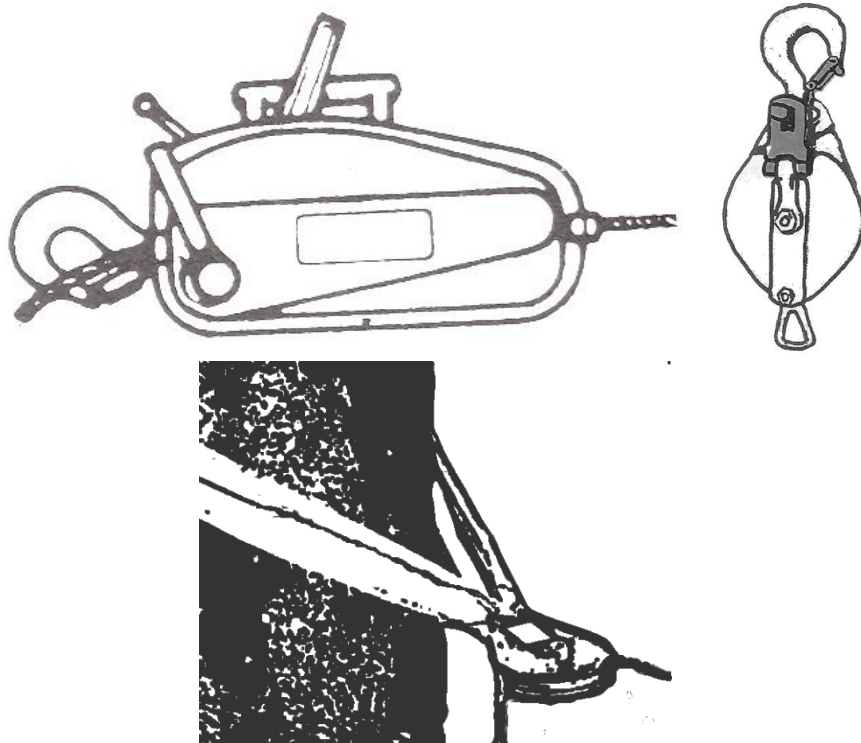
Tirfor da 1600 kg con carrucola apribile da 2000 kg e due cinghie tubolari lunghe 2,5-3 m da 2000 kg.
