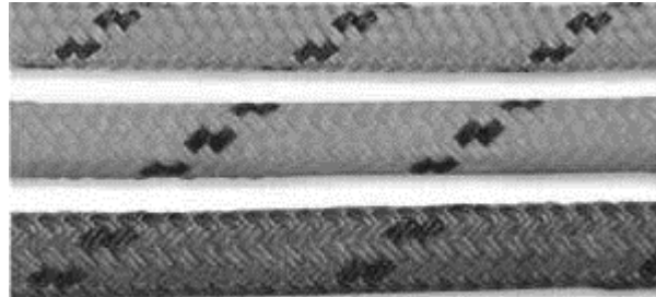
Corda da abbattimento da minimo 14,5 mm carico di rottura 62kN.
