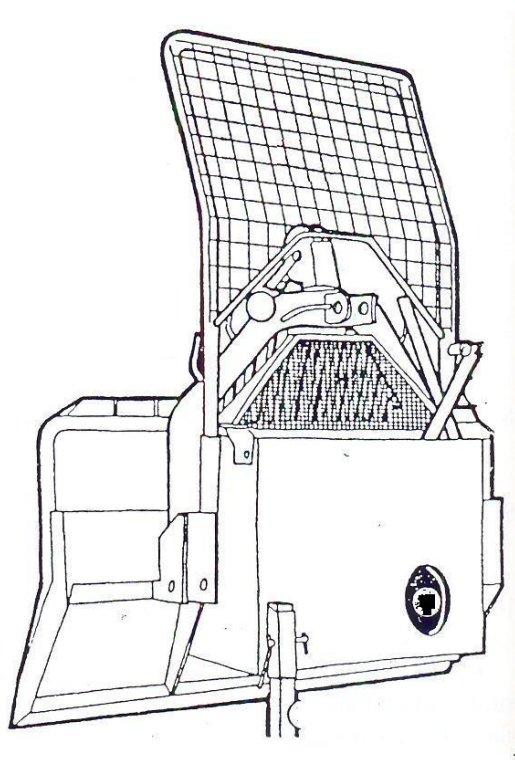
Verricello forestale con scudo e bocca di esbosco da 3500-4000 kg con fune da 10 mm e 3 ganci scorrevoli per altrettante catene.
